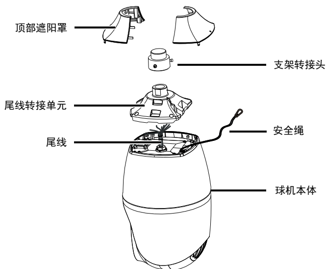
图2-1 设备组成（以红外球为例）
