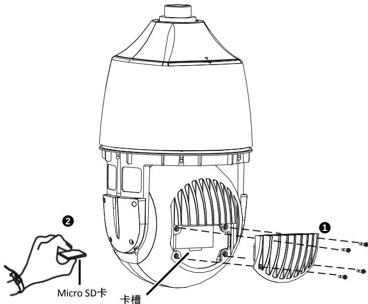
图2-3 安装 Micro SD 卡
